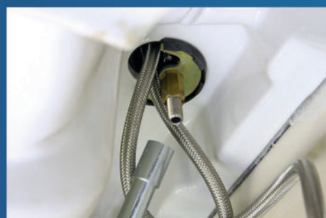
Betätigen der Armaturen-sicherungsschraube
